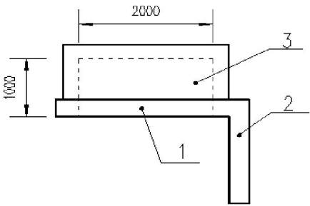
c) 俯视图
