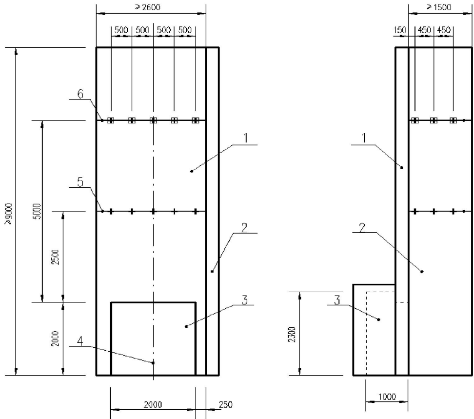
a) 正视图
