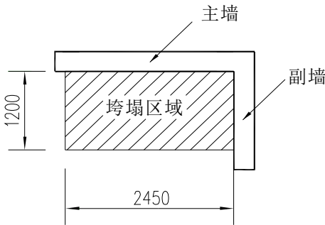
图 2 垮塌区域示意图
