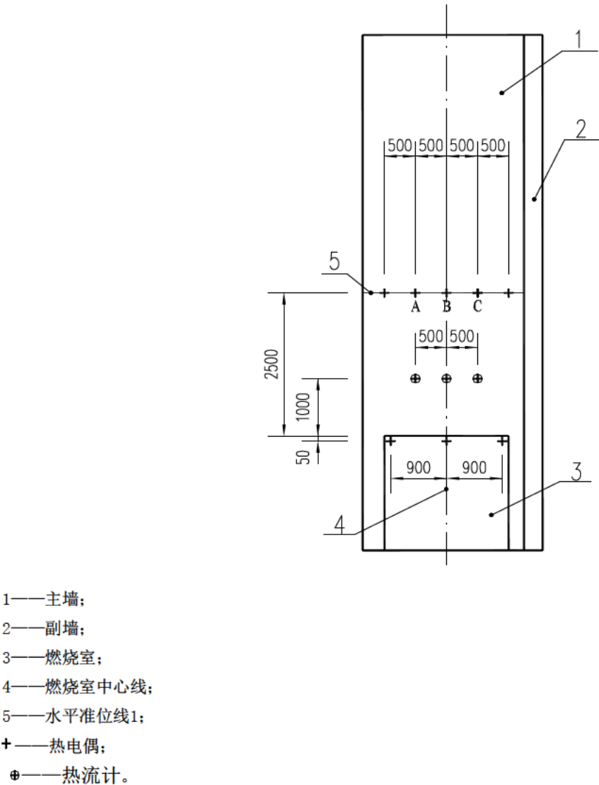
图A. 1 校准试验热流计和热电偶的布置位置
